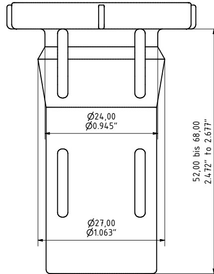
Clip-Stopfen IV mit Schwimmerschutz clip-in plug IV with float guard I4N260/330/420
