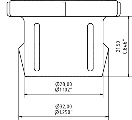
Clip-Stopfen IV für 4-Bajonett clip-in plug IV for 4-bayonet I4NV00
